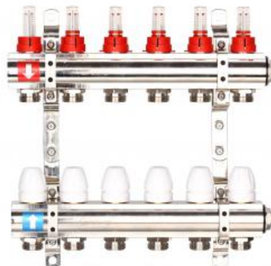
Коллектор регулируемый с расходомерами Gapp...
