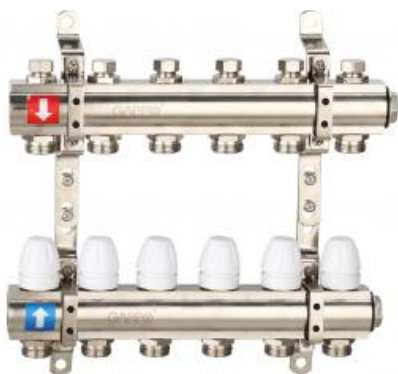
Коллектор регулируемый с запорными клапанам...
