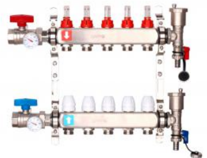
Коллектор регулируемый с расходомерами Gapp...
