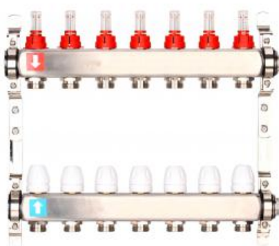
Коллектор регулируемый с расходомерами Gapp...
