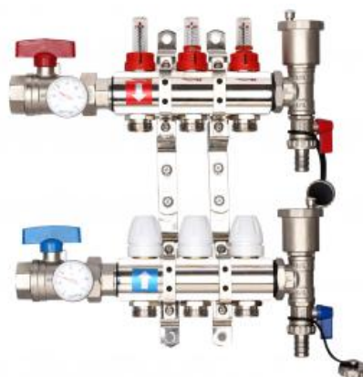
Коллектор регулируемый с расходомерами Gapp...
