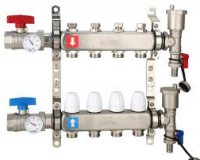
Коллектор регулируемый с запорными клапанам...
