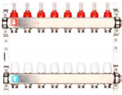
Коллектор регулируемый с расходомерами Gapp...
