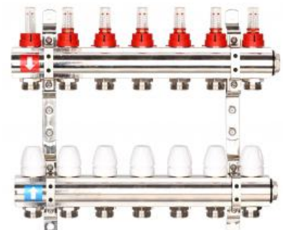
Коллектор регулируемый с расходомерами Gapp...
