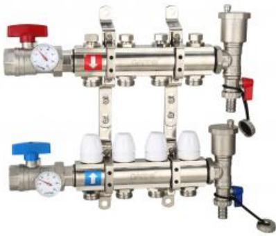
Коллектор регулируемый с запорными клапанам...
