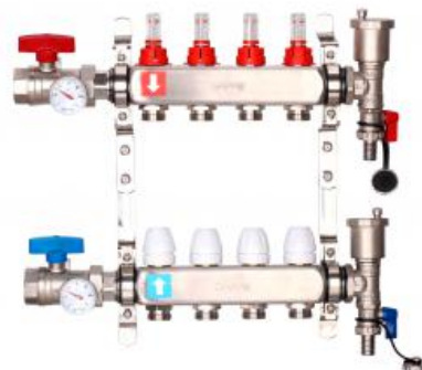
Коллектор регулируемый с расходомерами Gapp...
