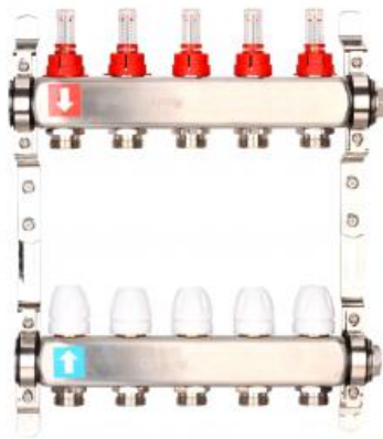
Коллектор регулируемый с расходомерами Garp...
