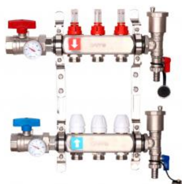
Коллектор регулируемый с расходомерами Garp...
