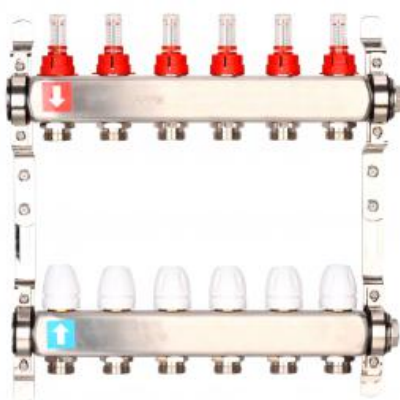
Коллектор регулируемый с расходомерами Garp...
